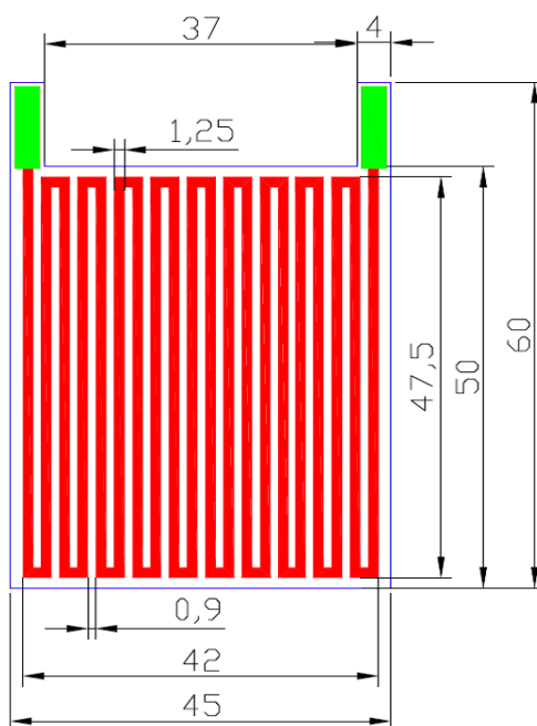
Рис. 1 –Топологическая схема резистивного слоя электронагревателя
