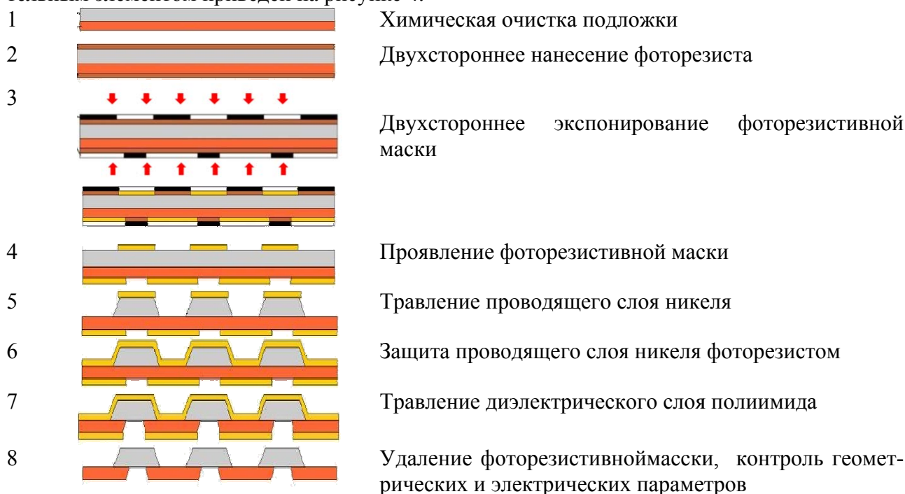
Рис.3 – Схематическая последовательность формирования проводящих и диэлектрических слоев плёночных нагревателей
